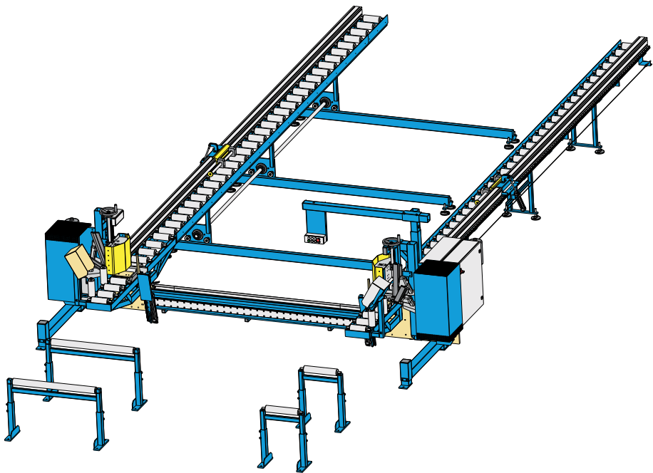
Riegelwerkstation FM1000TS
