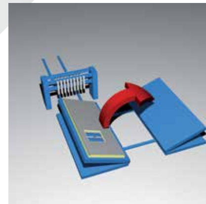
Wegklappbare Bolzen ermöglichen das Weiterführen der aufgerichteten Wand vom Einfach-System direkt in ein Lagersystem.
